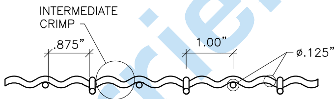
SECTION SCALE: 6"=1'-0"
